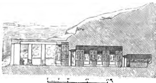
FIG. 241.—Longitudinal section, Derri ; from Horeau.
